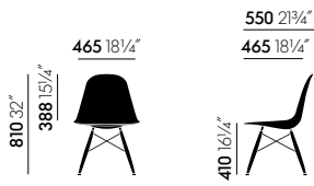
DSW, Holzuntergestell Ahorn mit Verstrebungen, nicht stapelbar, ohne Polster
