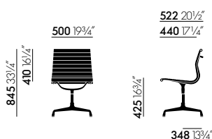
EA 101, nicht drehbar, ohne Armlehnen
