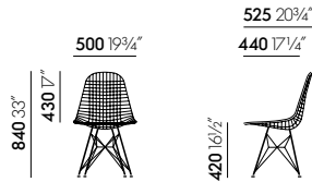
Wire Chair DKR, Vierbein-Drahtuntergestell mit Verstrebungen
