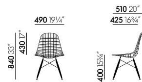
Wire Chair DKW, Holzuntergestell mit Verstrebungen aus Rundstahl
