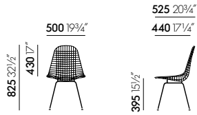
Wire Chair DKX, Vierbein-Stahlrohruntergestell
