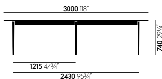
Tisch rechteckig, 3000 x 750 mm
