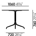
Tisch quadratisch, 750 x 750 mm
