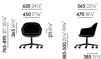
Softshell Chair, Fünfstern-Untergestell
