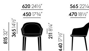
Softshell Chair, Vierbein-Untergestell
